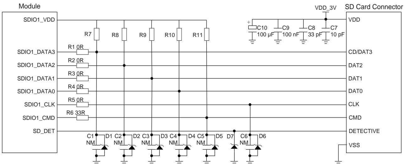
图 26: SD 卡接口电路参考设计
