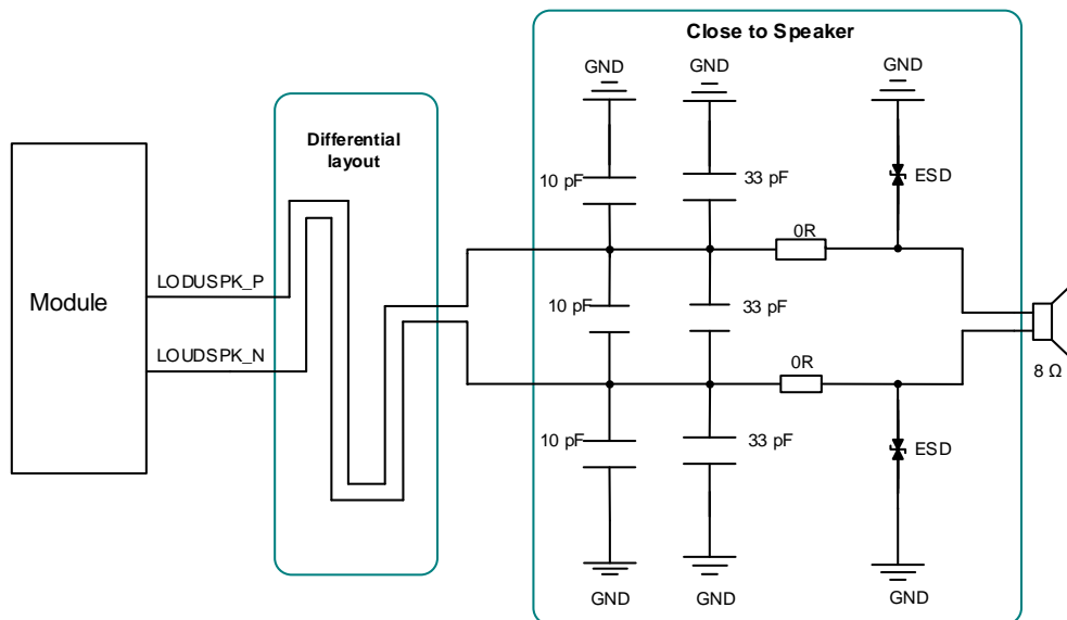
图 25: 扬声器输出参考电路
