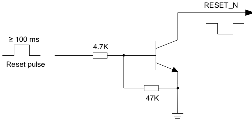
图 15: 开集驱动复位参考电路
