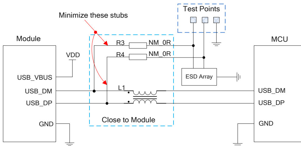
图 20: USB 接口参考设计
