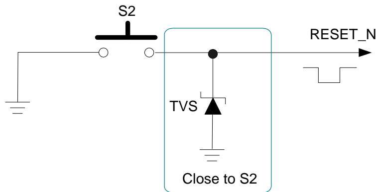
图 16: RESET_N 按键复位参考电路
