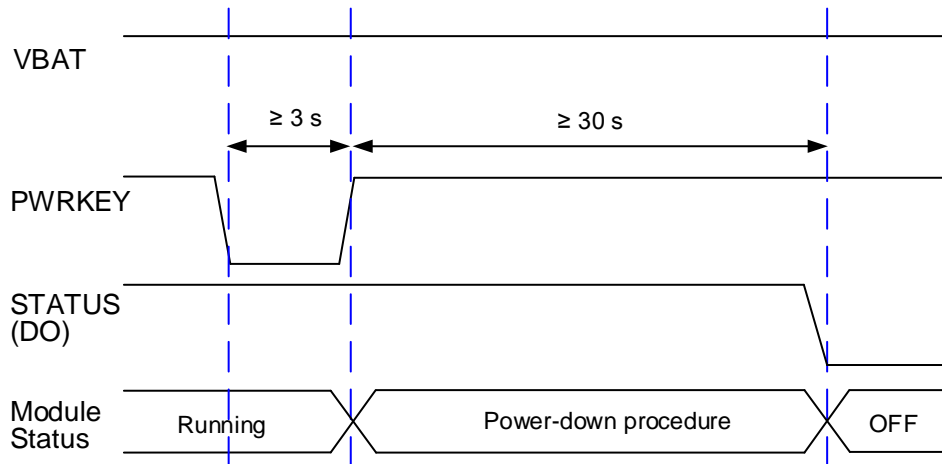
图 14：关机时序图
