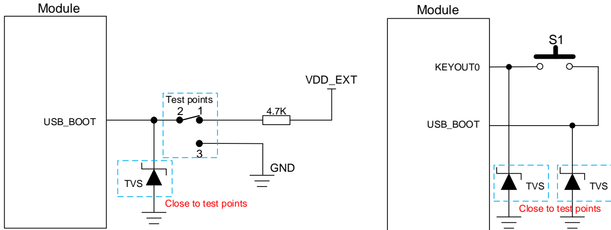
图 29: USB_BOOT 接口参考设计电路
