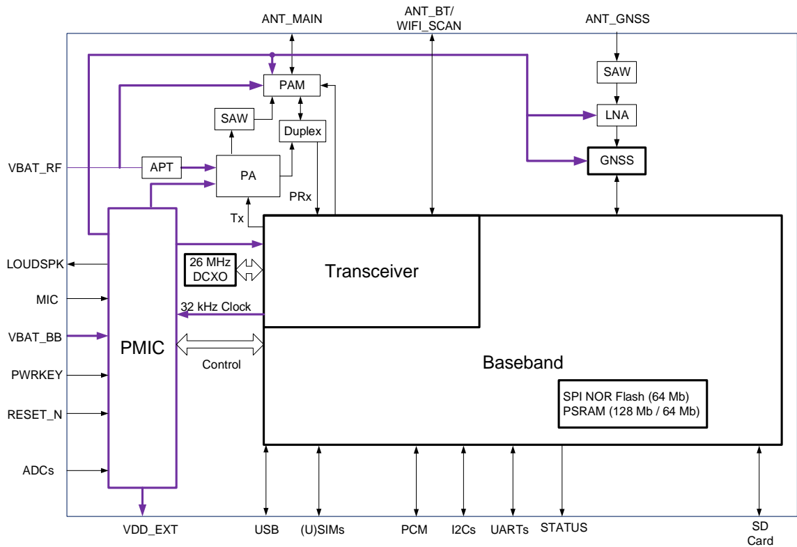
图 1：功能框图
