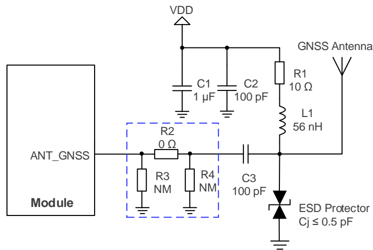
图 31: GNSS 天线参考电路
