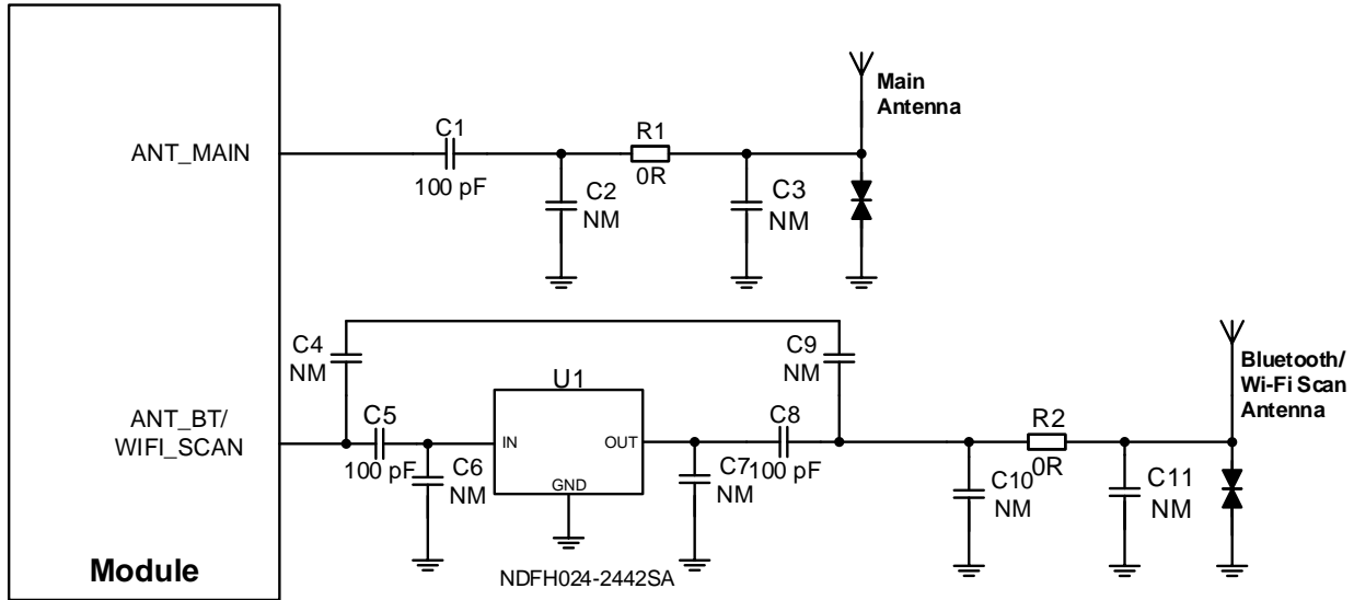
图 30: 射频参考电路
