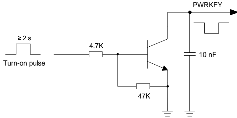
图 11：开集驱动开机参考电路
