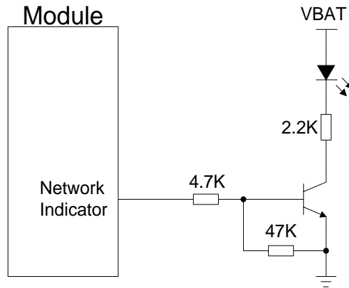
图 27: 网络状态指示参考电路
