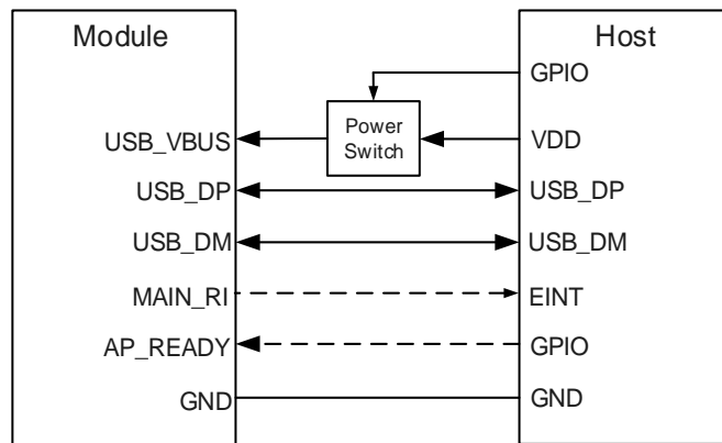
图 7：不支持 USB 挂起功能的睡眠应用
