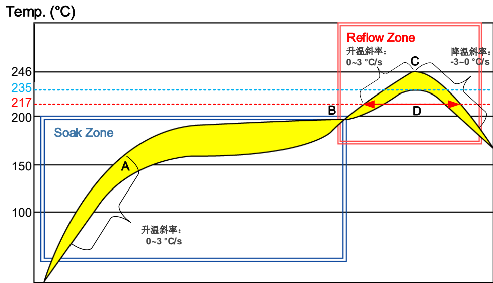
图 43: 推荐的炉温曲线图
