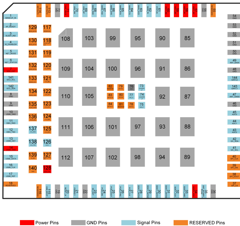
图 2: EC200U 系列模块引脚分配俯视图
