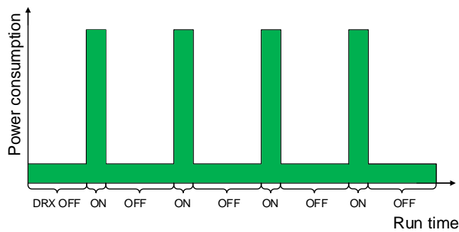
图 3：睡眠模式下模块功耗示意图
