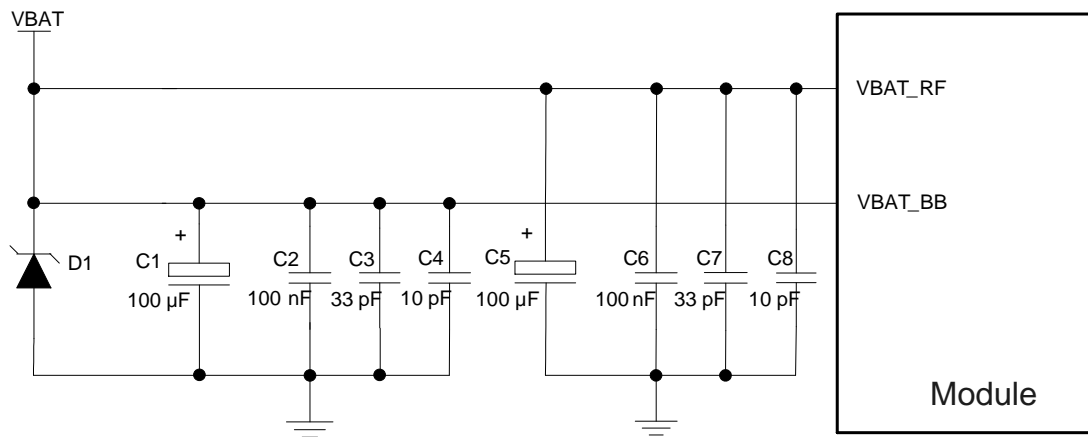
图 9：模块供电电路
