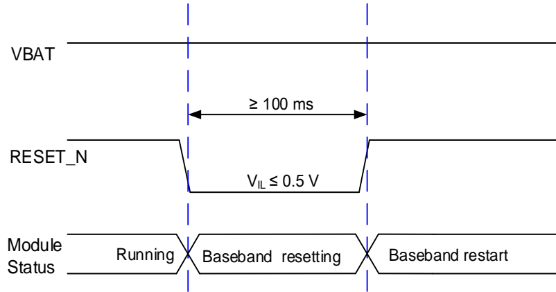
图 17: RESET_N 复位时序图
