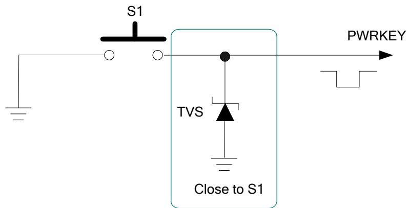
图 12：PWRKEY 按键开机参考电路
