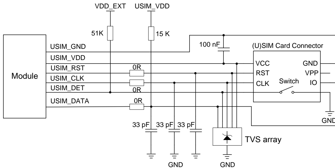
图 18: 8-pin (U)SIM 接口参考电路图
