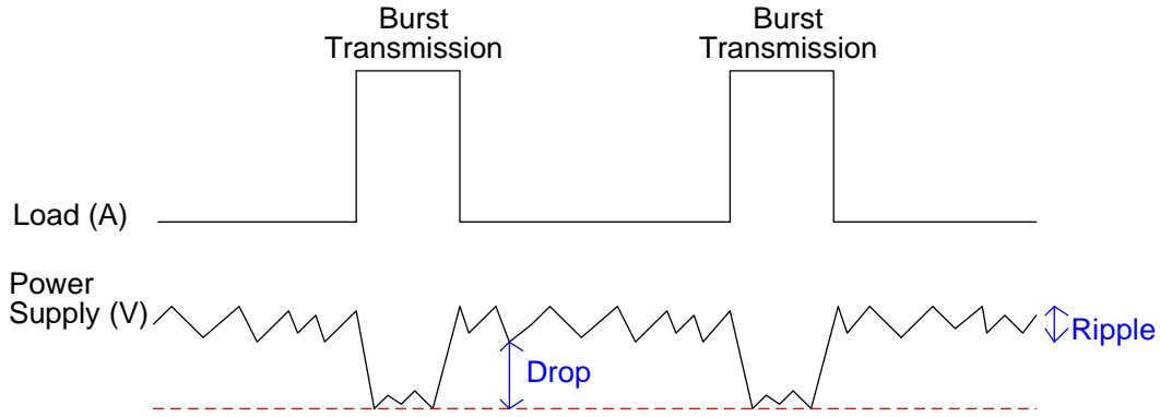
图 8：突发传输电源要求
