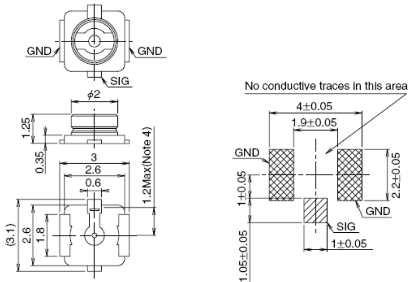
图 36: 天线座尺寸 (单位: mm)
