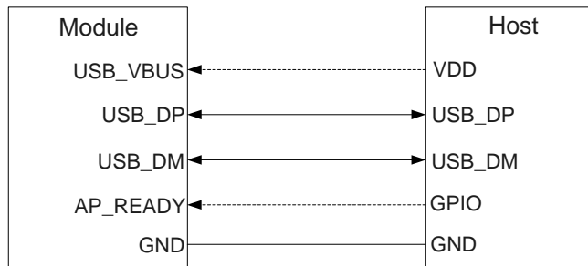
图 5: 带 USB 远程唤醒功能的睡眠应用
