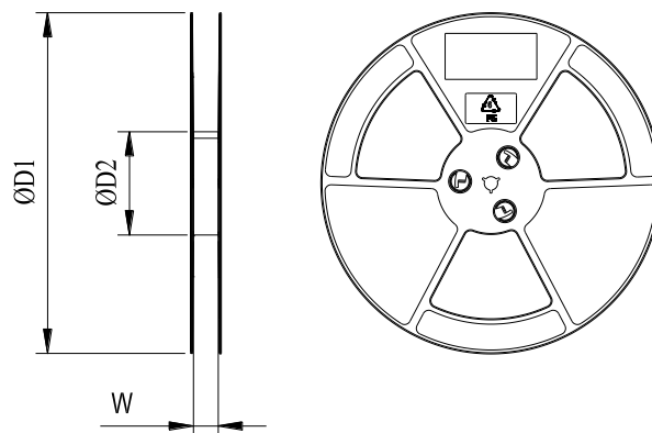
图 45: 胶盘尺寸图
