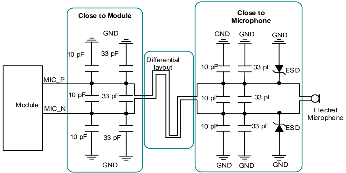
图 24: 麦克风接口参考电路
