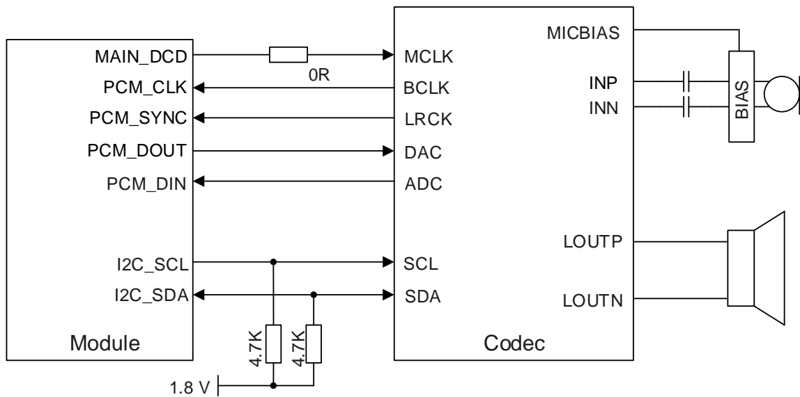
图 23: 外部 Codec 芯片 PCM 和 I2C 接口参考设计
