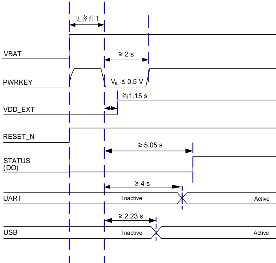
图 13: 开机时序图
