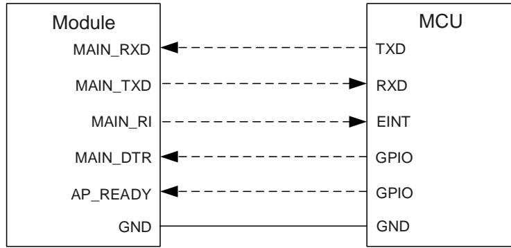
图 4: UART 睡眠应用
