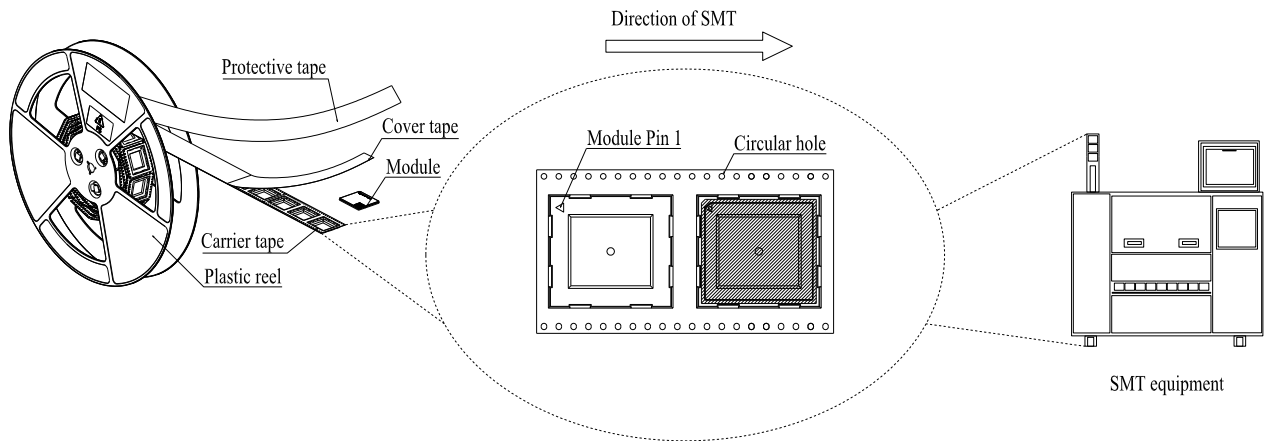
图 46: 贴片方向
