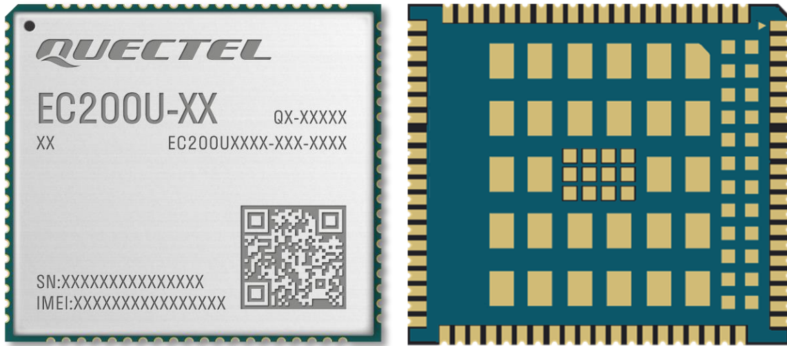
图 42: 模块俯视图和底视图
