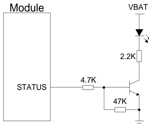
图 28: STATUS 参考电路
