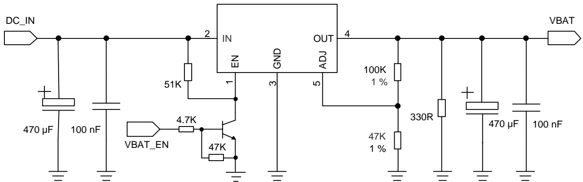
图 10: 供电输入参考设计
